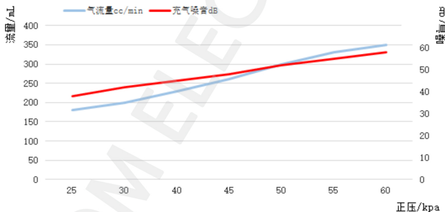
特性曲线图 Characteristic curve: 流量和噪音变化
